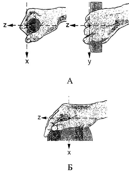
Рис. П 7.2. Направление осей при измерениях локальной вибрации А — при охвате цилиндрических, торцовых и близких к ним поверхностей Б — при охвате сферических поверхностей
